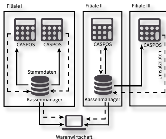
Abb. Beispielaufbau
